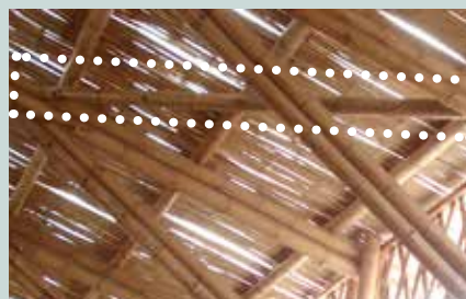
Tirante que asegura la rigidez del techo
